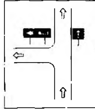
Şekil: Tek yönlü ayrılmalarında B-16b kullanımı
