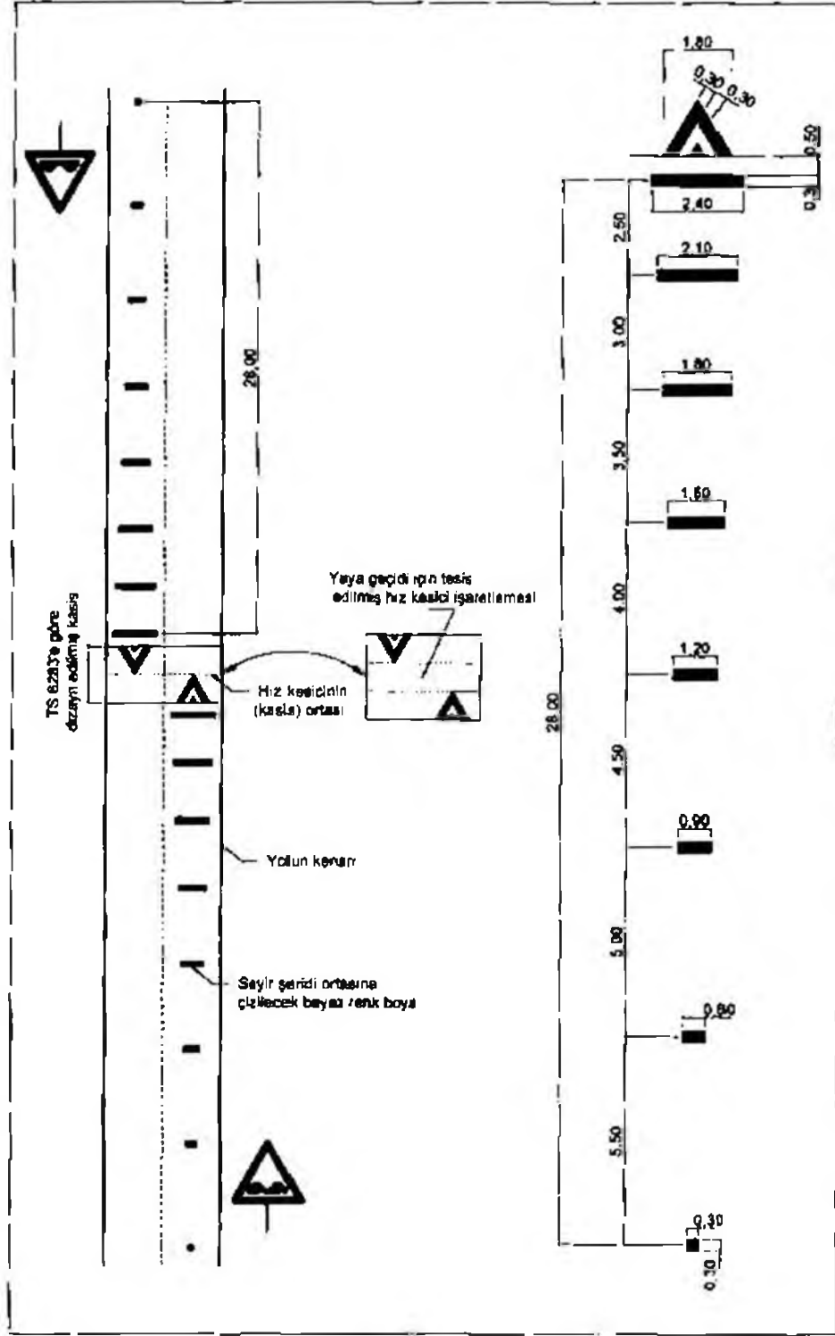
Şekil: Hız kesici tümseklerin (kasislerin) işaretlenmesi
